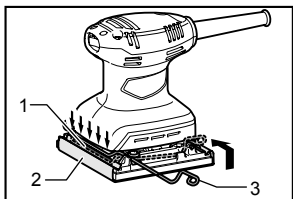
1. Parte (pieza) de sujeción 2. Papel abrasivo 3. Palanca
