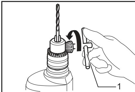
► 1. Chuck key
