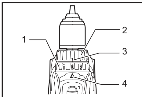
► 1. Bague de changement de mode d'action 2. Bague de réglage 3. Graduation 4. Flèche
