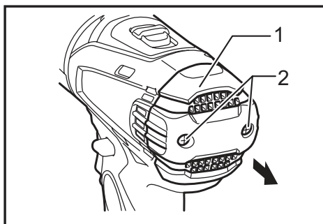
► 1. Cubierta trasera 2. Tornillo
