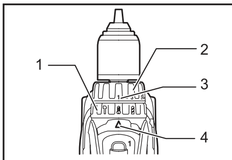
► 1. Bague de changement de mode d'action 2. Bague de réglage 3. Graduation 4. Flèche
