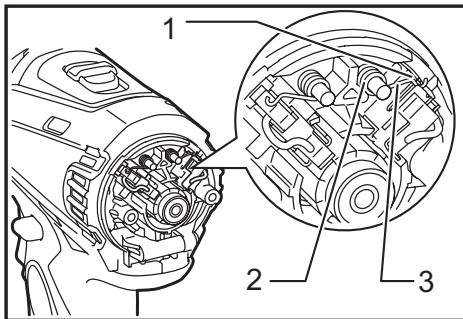
► 1. Parte rebajada 2. Resorte 3. Brazo
