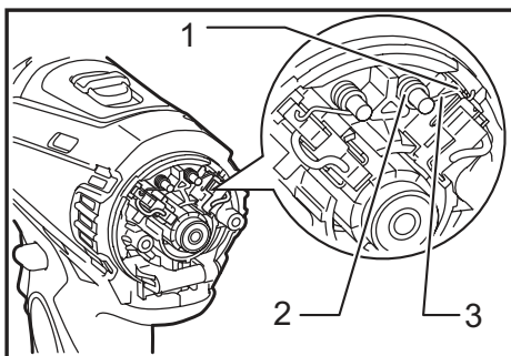
► 1. Partie encastrée 2. Ressort 3. Bras
