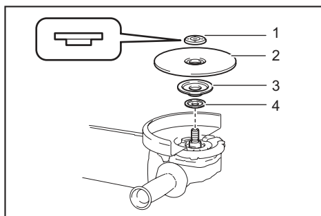
► 1. Contratuerca 2. Disco flexible 3. Plato de respaldo 4. Brida interior
