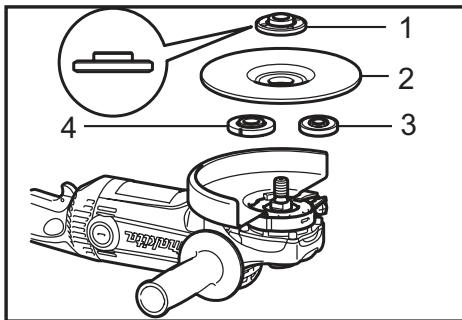
► 1. Contratuercas 2. Disco con el centro rebajado 3. Brida interior 4. Brida superior
