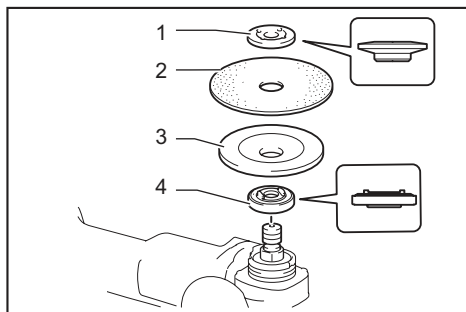
► 1. Contratuercas para lijar 2. Disco abrasivo 3. Plato de caucho 4. Brida interior
