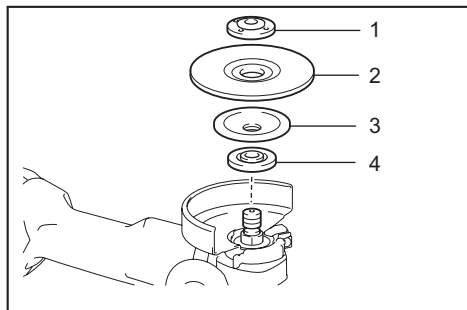
► 1. Contratuera 2. Disco flexible 3. Plato de respaldo 4. Brida interior
