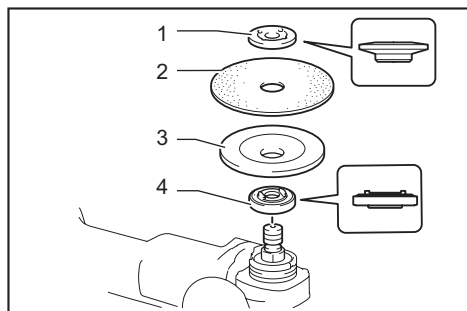
► 1. Contratuera para lijar 2. Disco abrasivo 3. Plato de caucho 4. Brida interior
