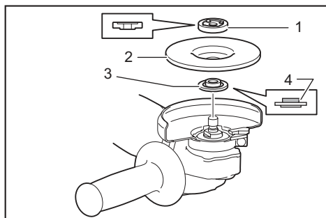
► 1. Contratuera 2. Muela de centro hundido 3. Brida interior 4. Parte de montaje
