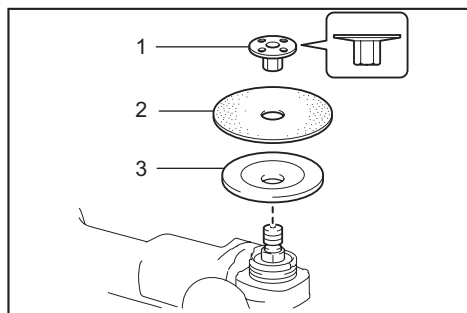
► 1. Contratuera para lijar 2. Disco abrasivo 3. Plato de caucho
