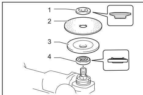
► 1. Contratuercas para lijar 2. Disco abrasivo 3. Plato de caucho 4. Breda interior
