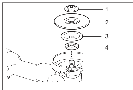
► 1. Contratuercas 2. Disco flexible 3. Plato de respaldo 4. Breda interior
