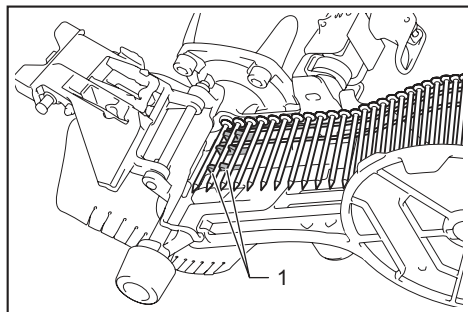
► 1. Feed Claw
